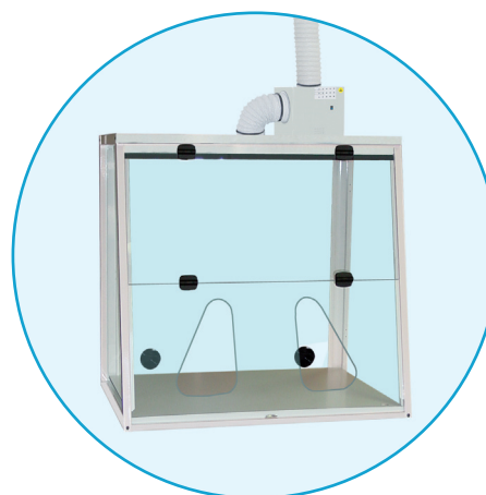
▲ BH09D + BB09 + caisson de ventilation modèle CDV-A + 2 kits de raccordement pour caisson référence KRC
